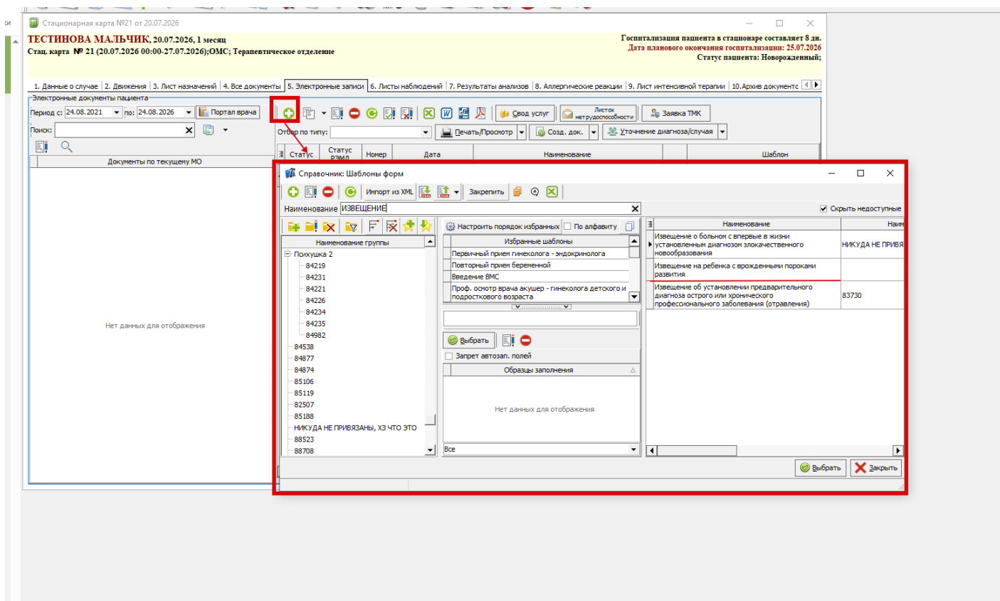
Рисунок 4 – Выбор шаблона.
