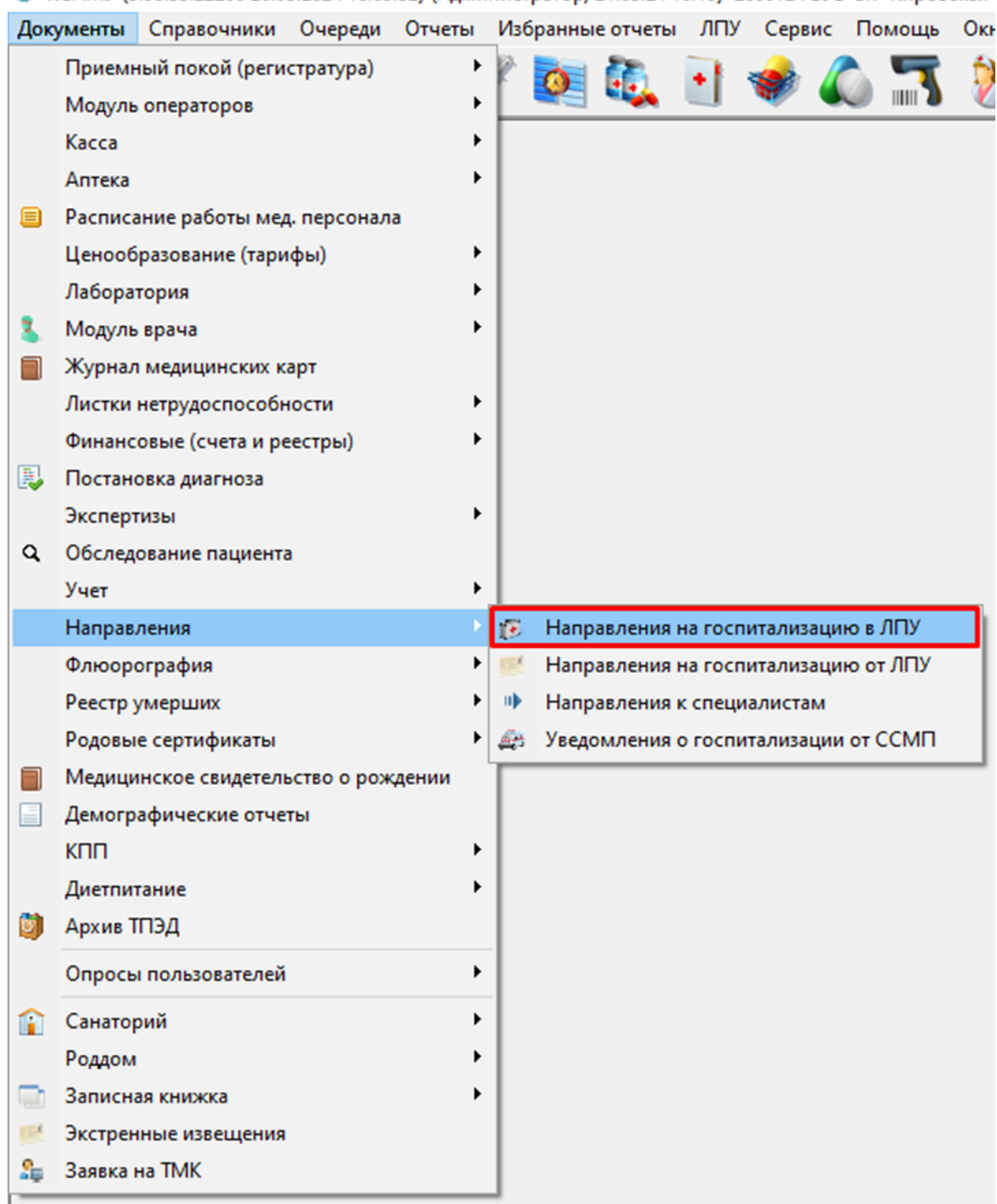
Рисунок 6 - Журнал направлений
