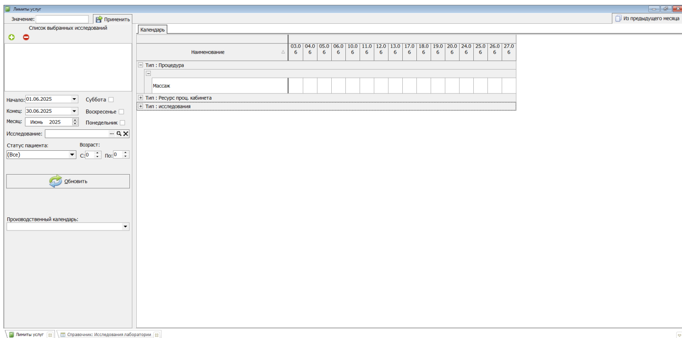
Рисунок 2 - Заполнение документа
