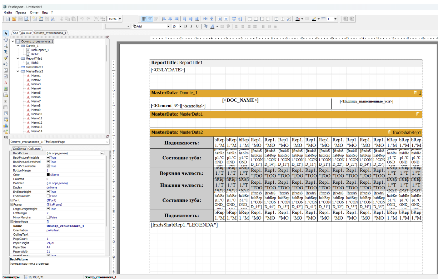
Рисунок 4 - Пример размещения зубной формулы в редакторе печатных форм
